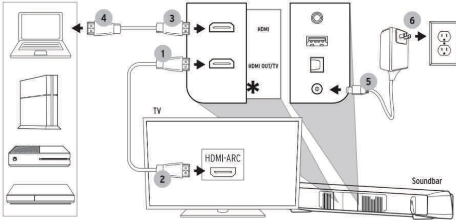
Verkabelung von ARC zu TV
